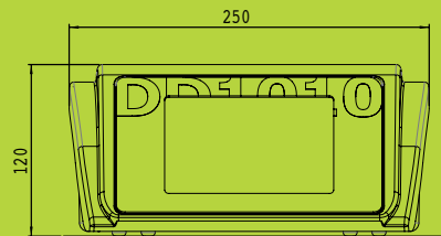
DD1010 versione da tavolo
