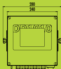
DD1010i fissaggio a parete
