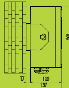
DD1010i fissaggio a parete
