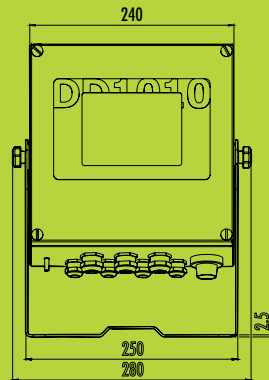
DD1010i versione da tavolo
