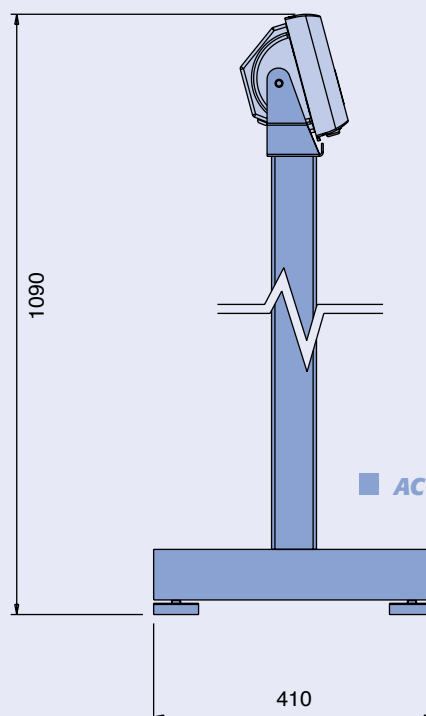
Colonna con piedistallo per collegamento a piattaforma di pesatura
