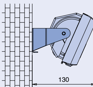
D 70 E versione per fissaggio a parete
